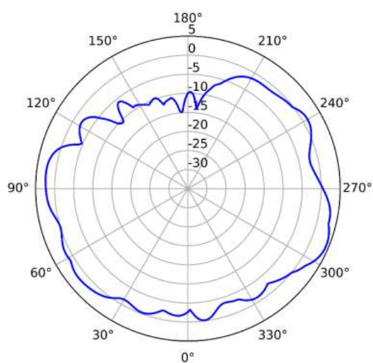
6GHz (Vertical)
